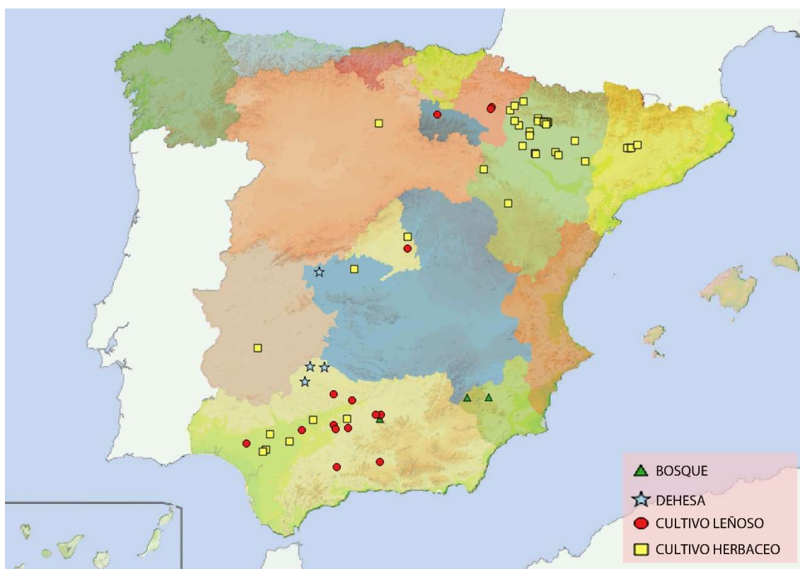
Figura 13: Ubicación de los estudios a escala local revisados.
