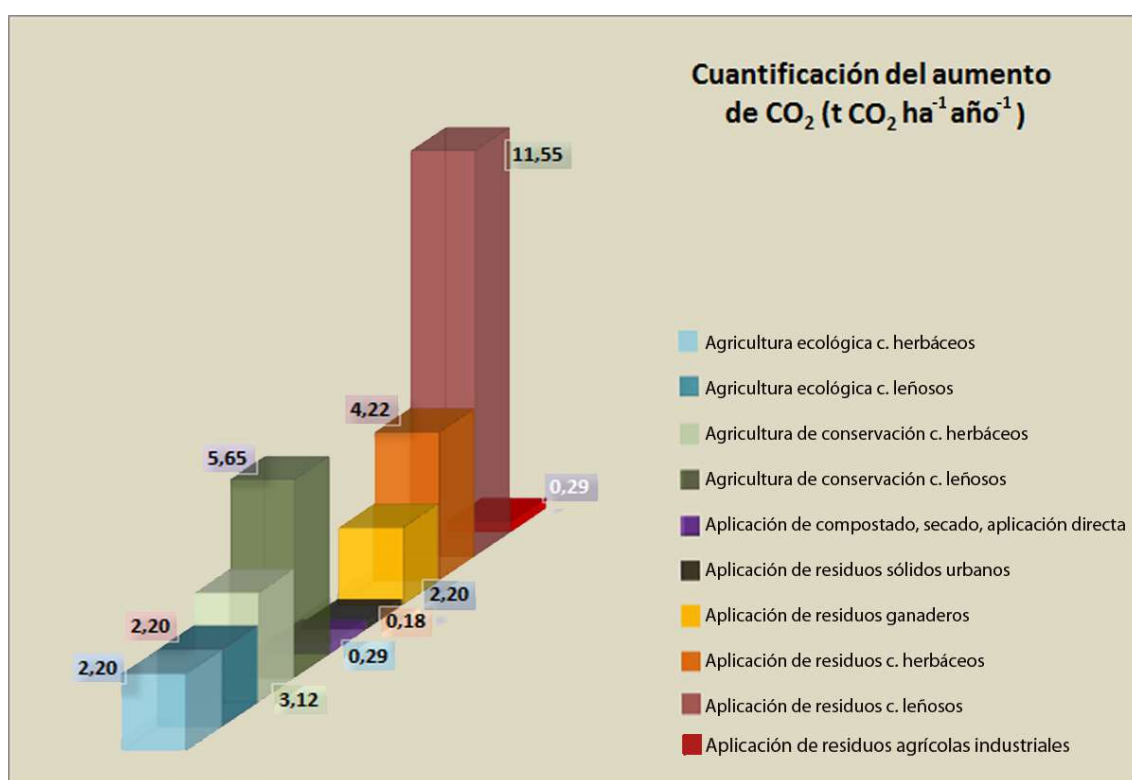
Figura 1. Cuantificación del aumento de emisiones CO 2 capturadas en suelo debido a la aplicación de diferentes medidas (t CO 2 ha -1 año -1 ).
