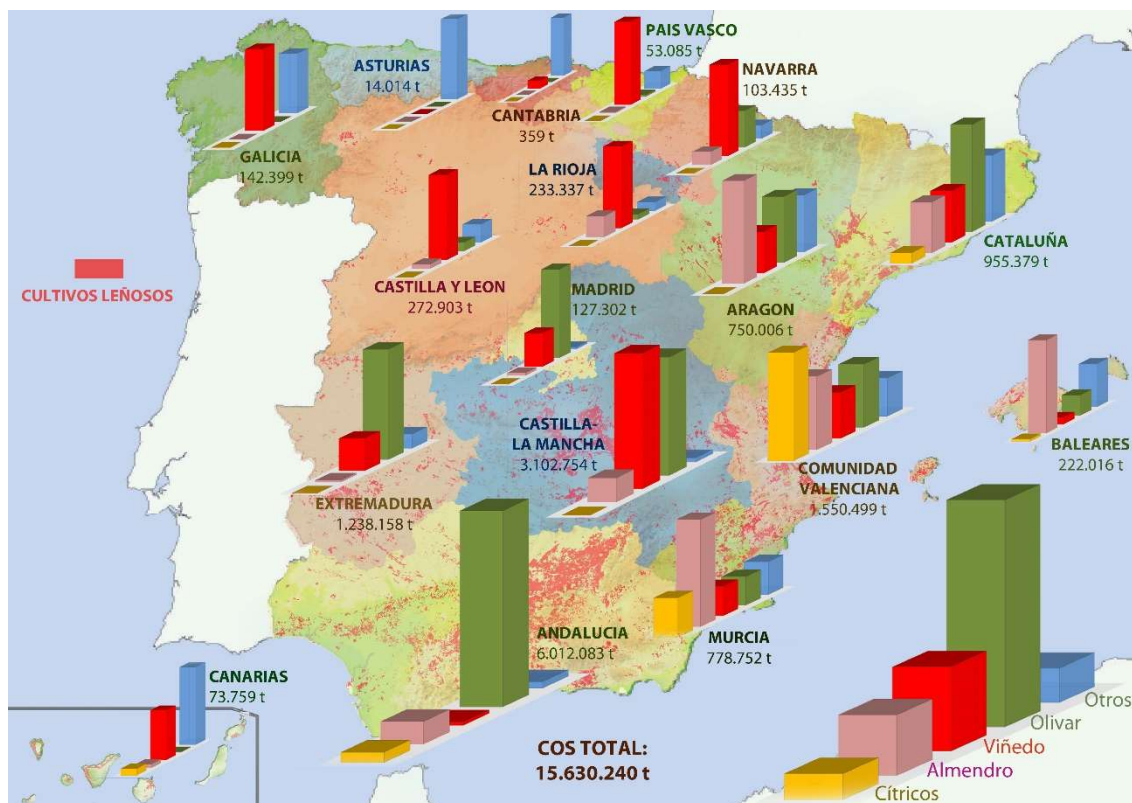
Figura 2. Potencial de fijación de COS partir de la aplicación de restos de poda en los principales cultivos leñosos y en la totalidad de la superficie con cultivos leñosos (entre paréntesis).
