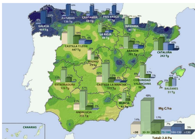
Figura 2. Contenido de carbono orgánico del suelo en España y en cada Comunidad Autónoma.
