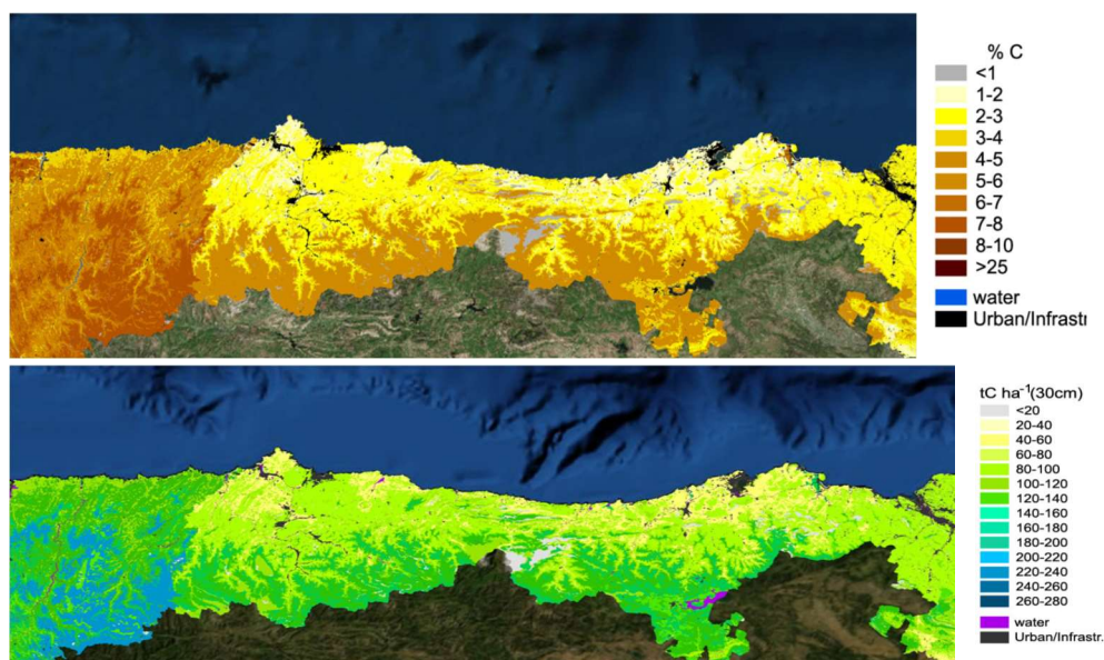
Figura 9. Contenido de COS en los 30 primeros cm de suelo de Asturias y Cantabria. Fuente: Calvo de Anta et al. (1015)
