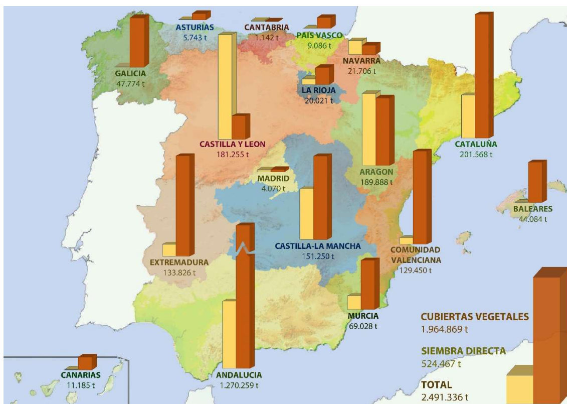
Figura 2. Estimación de la cantidad de COS almacenado actualmente en los suelos en cultivos leñosos (cubiertas vegetales) y cultivos herbáceos (siembra directa) debido a la Agricultura de Conservación.
