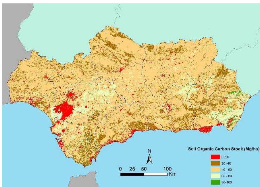
Figura 12. Contenido de COS en los 75 primeros cm de suelo en Andalucía. Fuente: Muñoz-Rojas et al. (2012).
